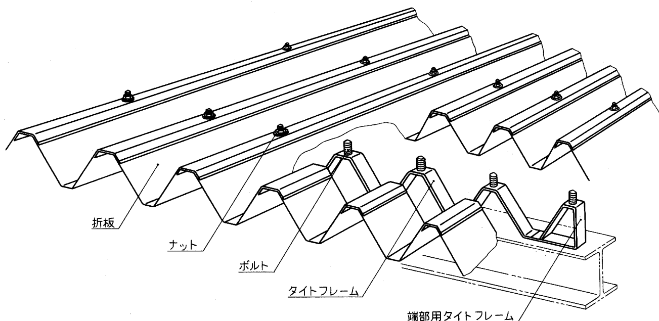
図1 重ね形折板屋根の例
