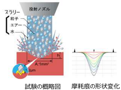
試験の概略図
