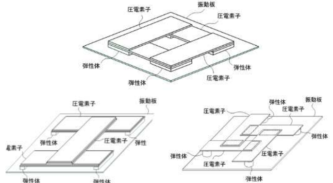
圧電素子アレイを用いた参考例
