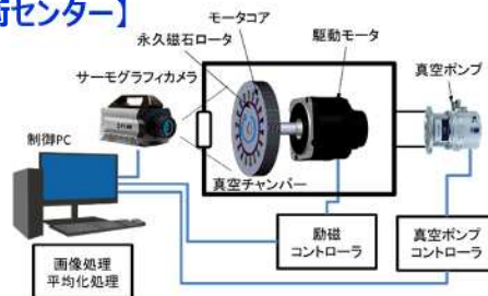
【装置構成概略】
