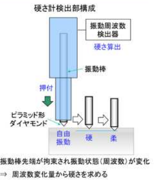
超音波接触インピーダンス(UCI)硬さ測定方法のイメージ
