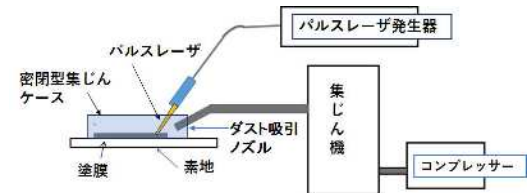
パルスレーザー塗膜除去装置の構成概要
