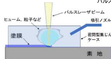
パルスレーザーアブレーションによる塗膜除去のイメージ
